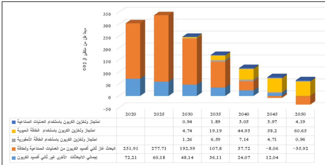
الشكل رقم (57): انبعاث ثنائي أكسيد الكربون وفق سيناريو صافي الانبعاثات صفر بحلول عام 2050
