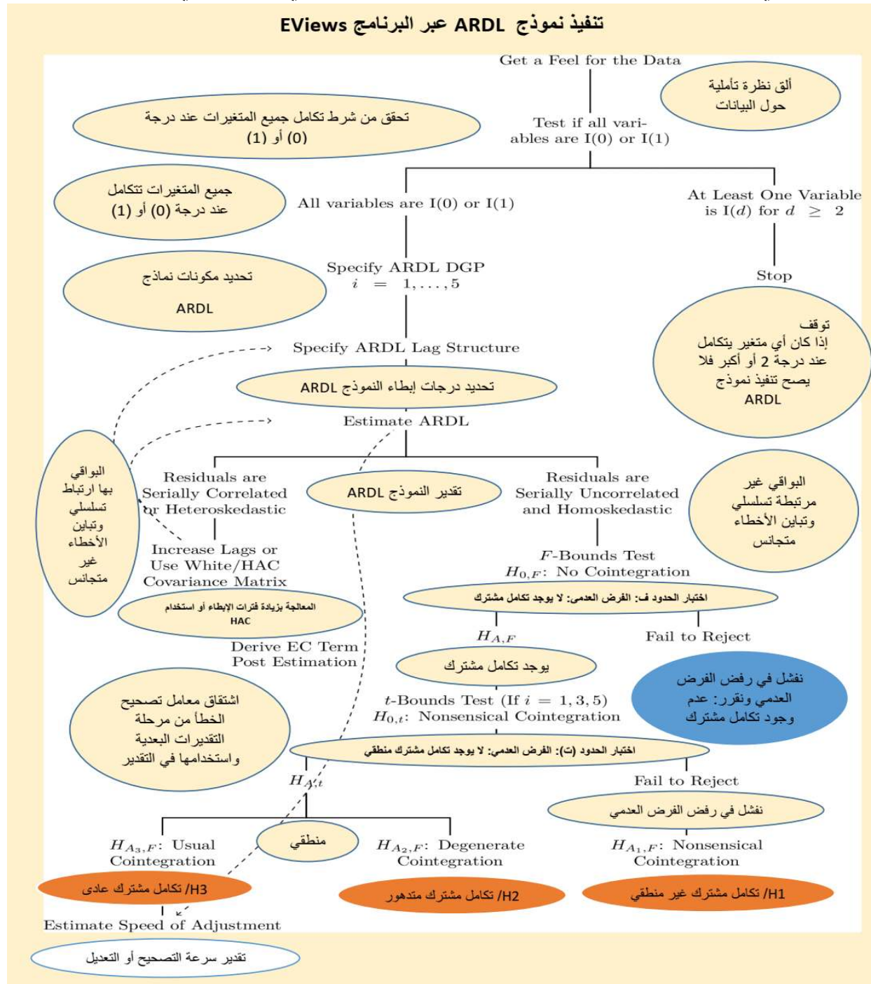
شكل رقم 03 - 07: خطوات تنفيذ نموذج ARDL
