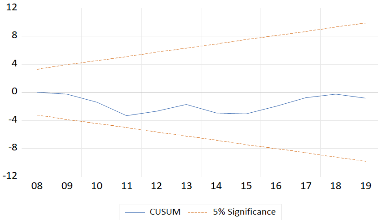
شكل رقم 03-14 : اختبار CUSUM لنموذج X
