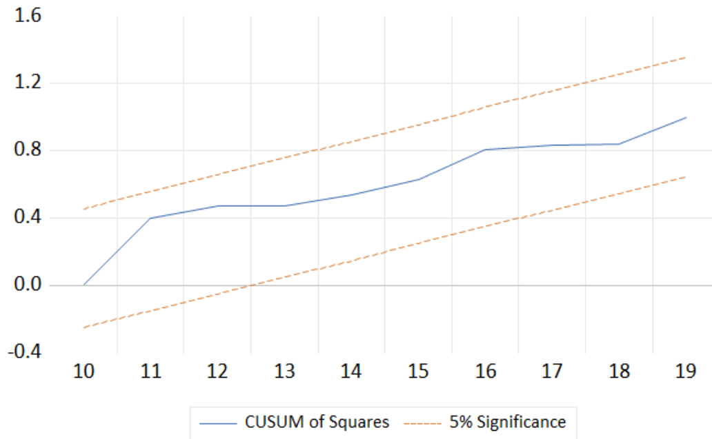
شكل رقم 03-13 : اختبار CUSUM SQ لنموذج IPH
