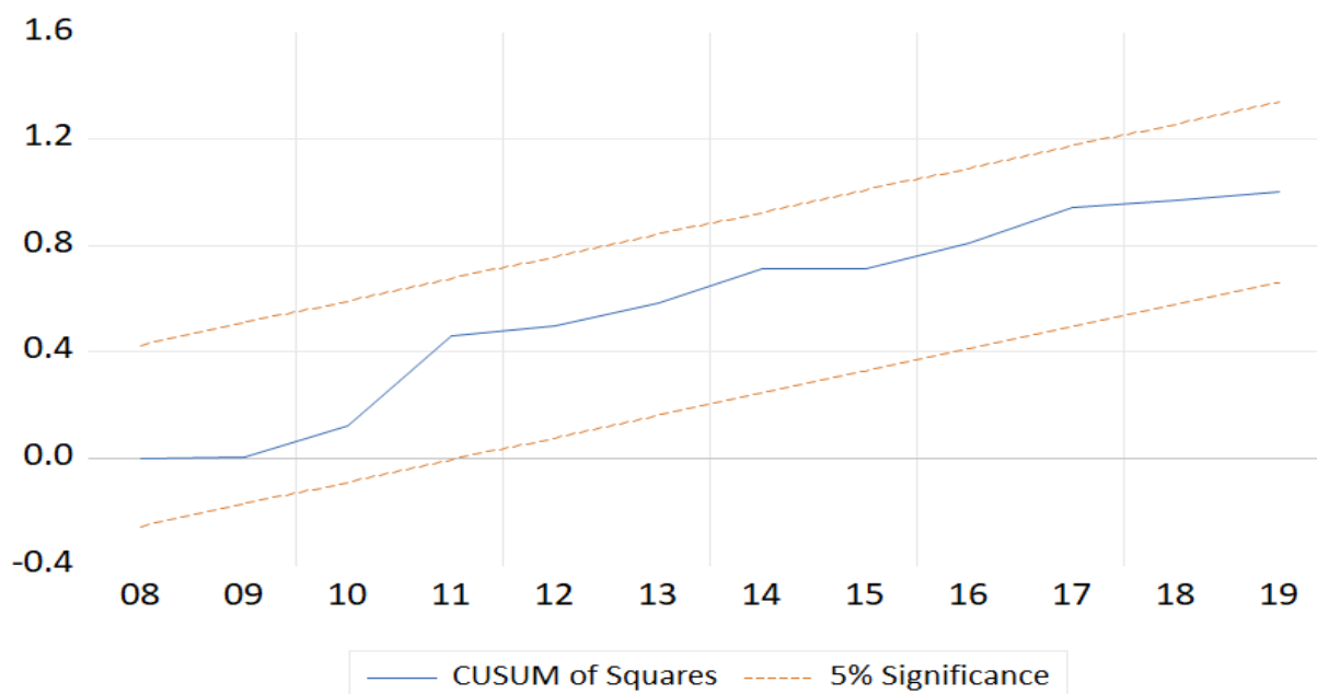
شكل رقم 03-15 : اختبار CUSUM SQ لنموذج X
