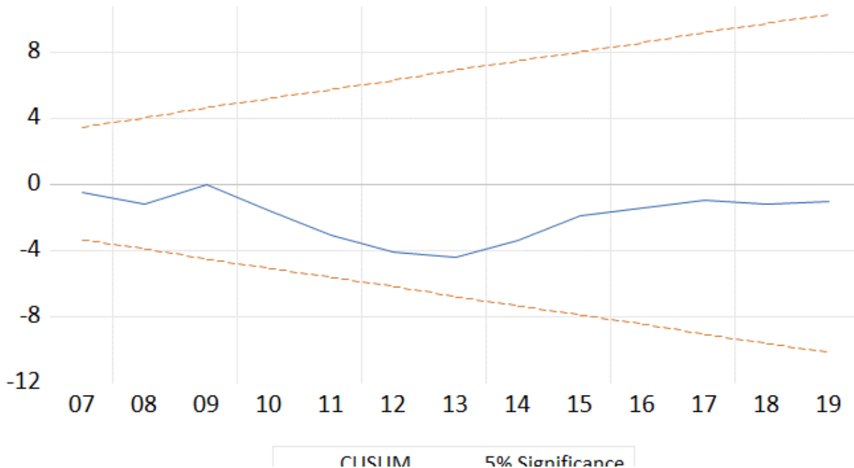
شكل رقم 10-03: اختبار CUSUM لنموذج IM
