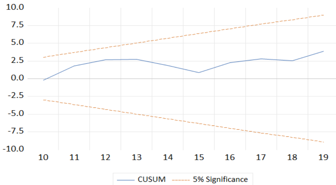
شكل رقم 12-03 : اختبار CUSUM لنموذج IPH
