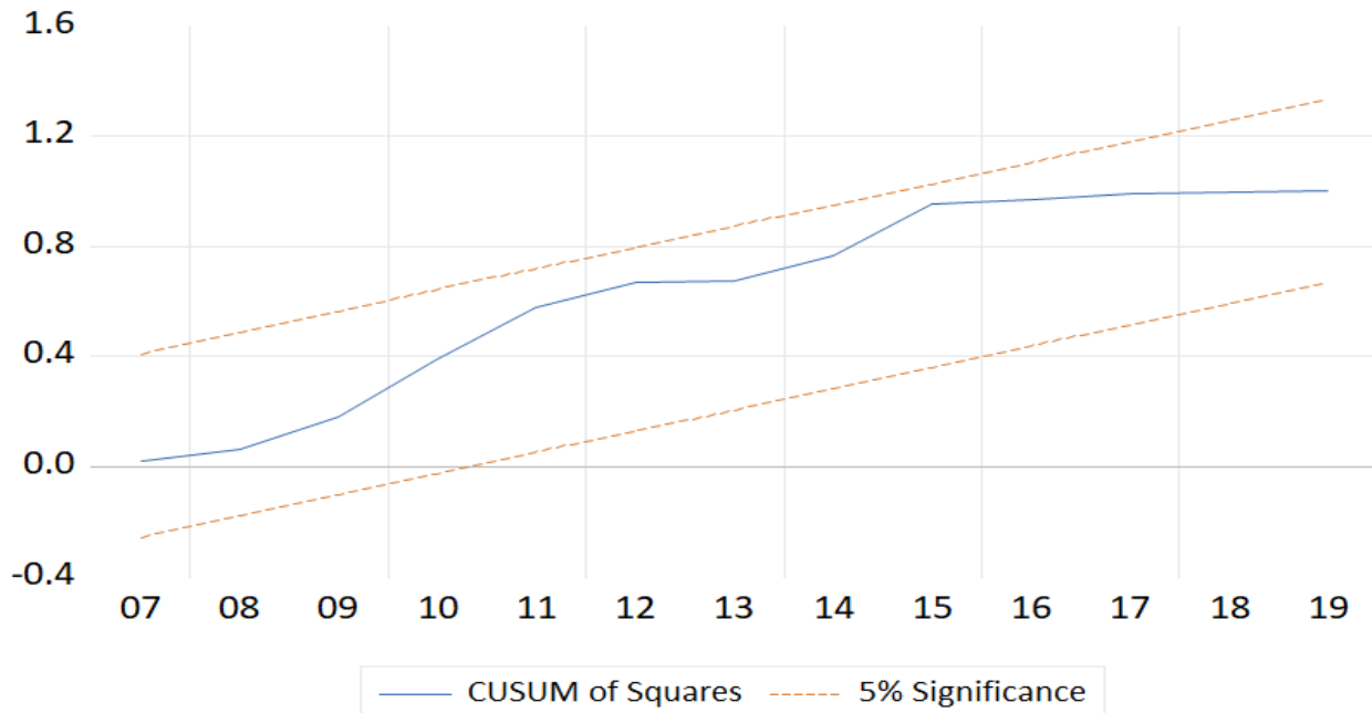
شكل رقم 11-03: اختبار CUSUM SQ لنموذج IM
