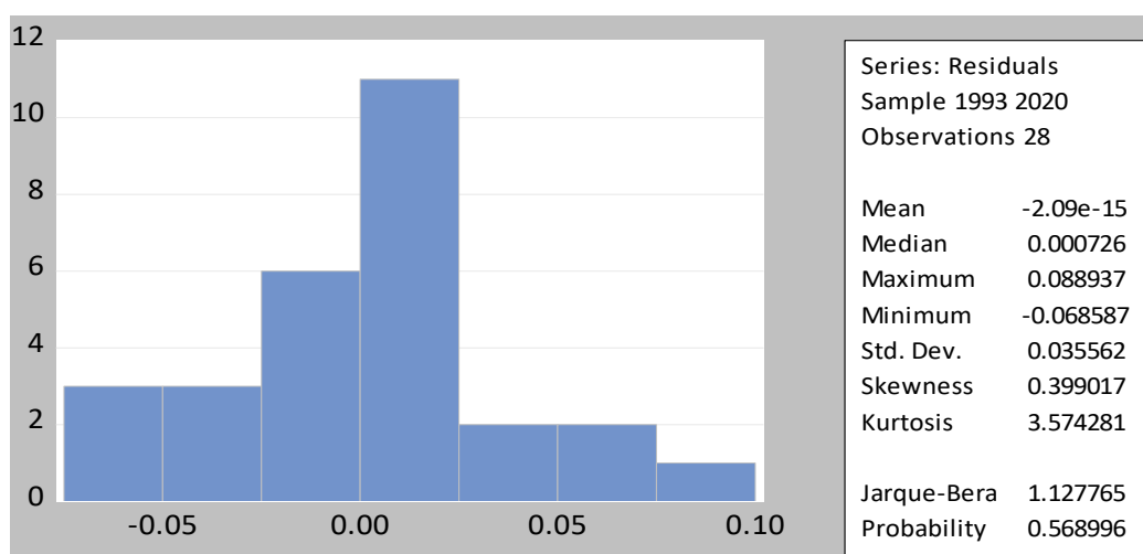
الشكل رقم 04 – 11 : التوزيع الطبيعي للبواقي
