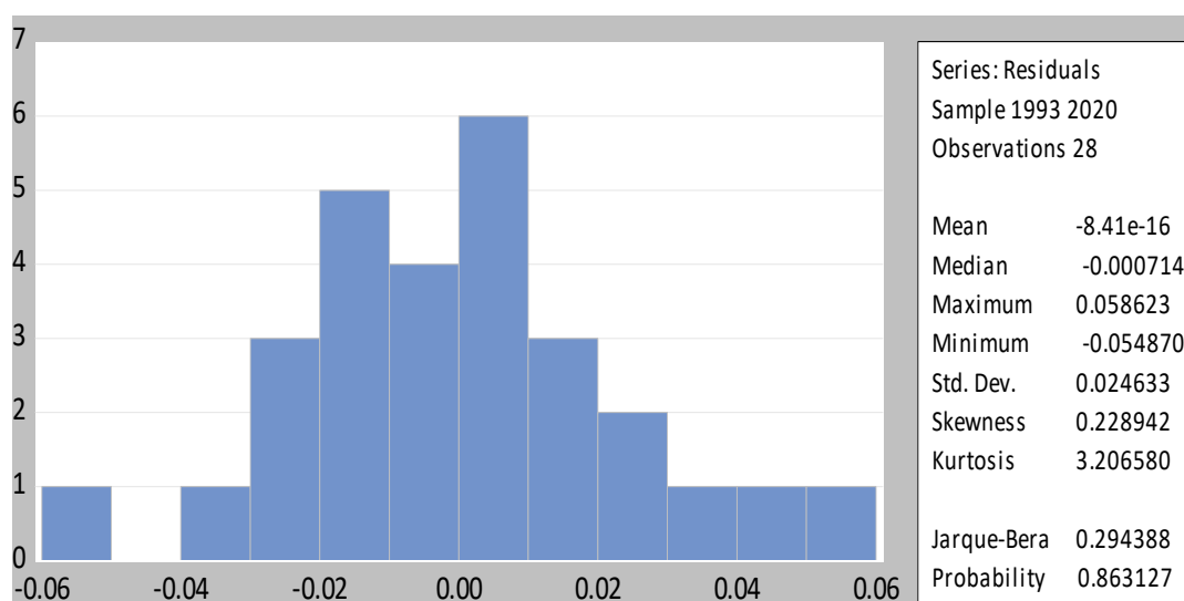
الشكل رقم 04 – 07 : التوزيع الطبيعي للبواقي
