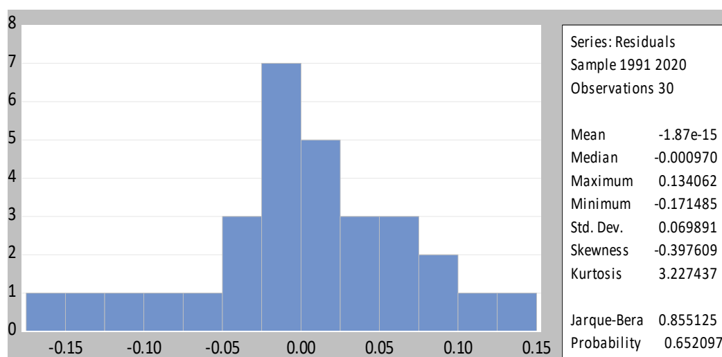
الشكل رقم 04 – 03 : التوزيع الطبيعي للبواقي
