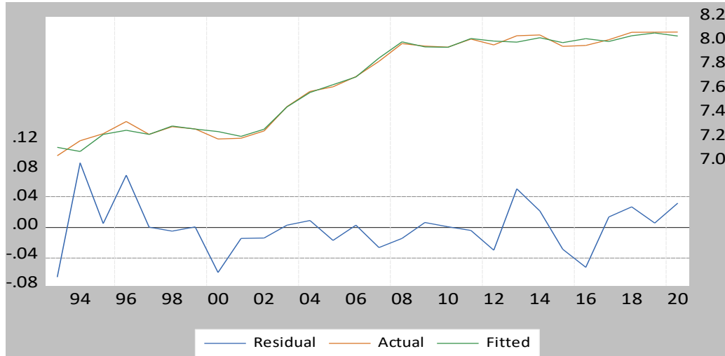
الشكل رقم 04-10: تقارب القيم الحقيقية والمقدرة، والبقايا
