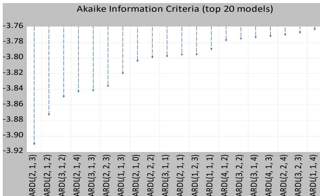
الشكل رقم 04 – 05 : نتائج اختبار فترات الابطاء المثلى
