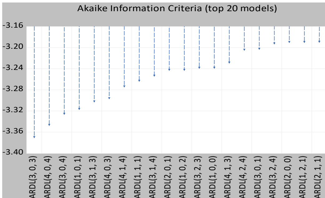
الشكل رقم 04 – 09 : نتائج اختبار فترات الابطاء المثلى
