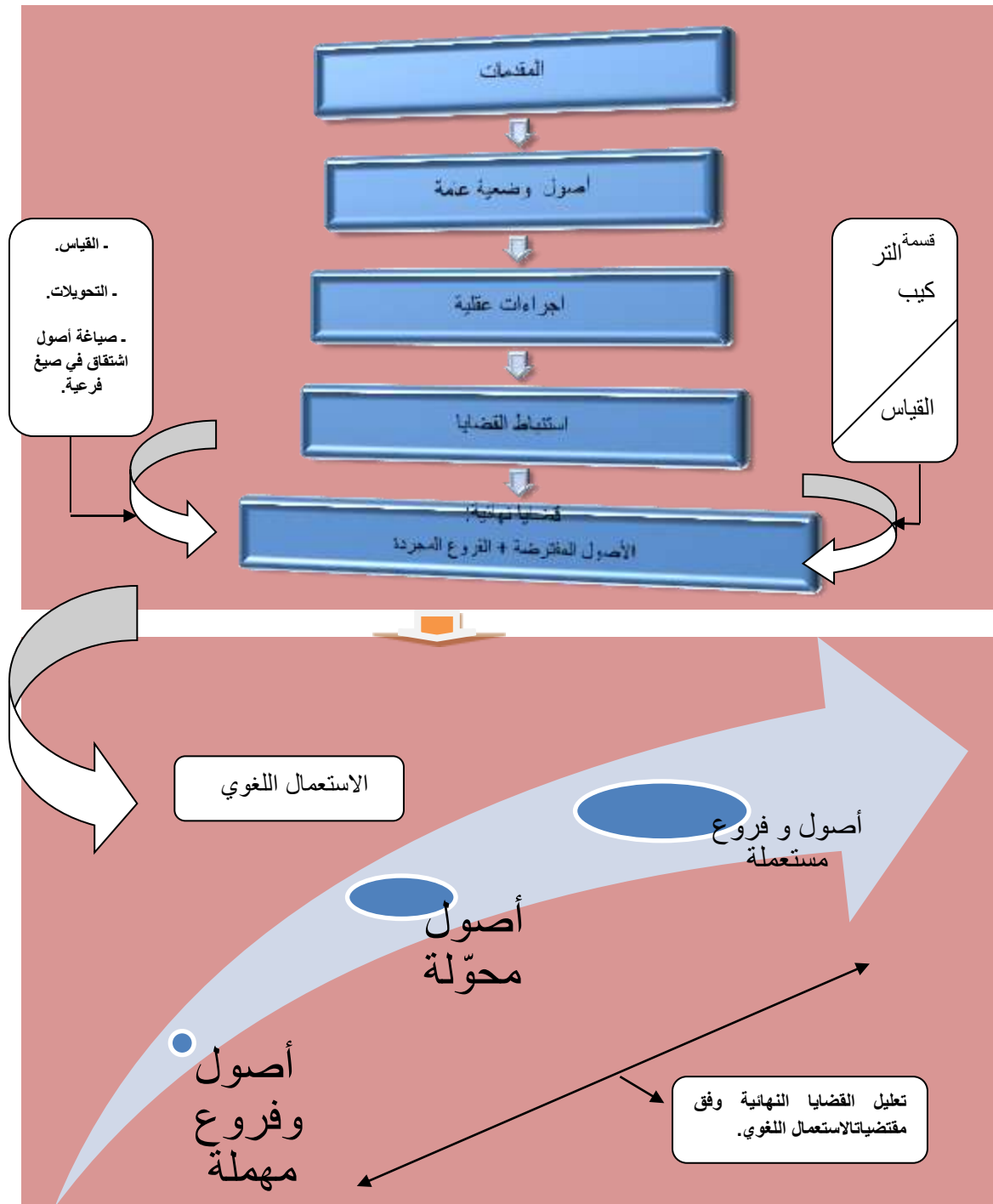
الشكل 34: مجريات المسلك الثاني للنسق الاستنباطي
